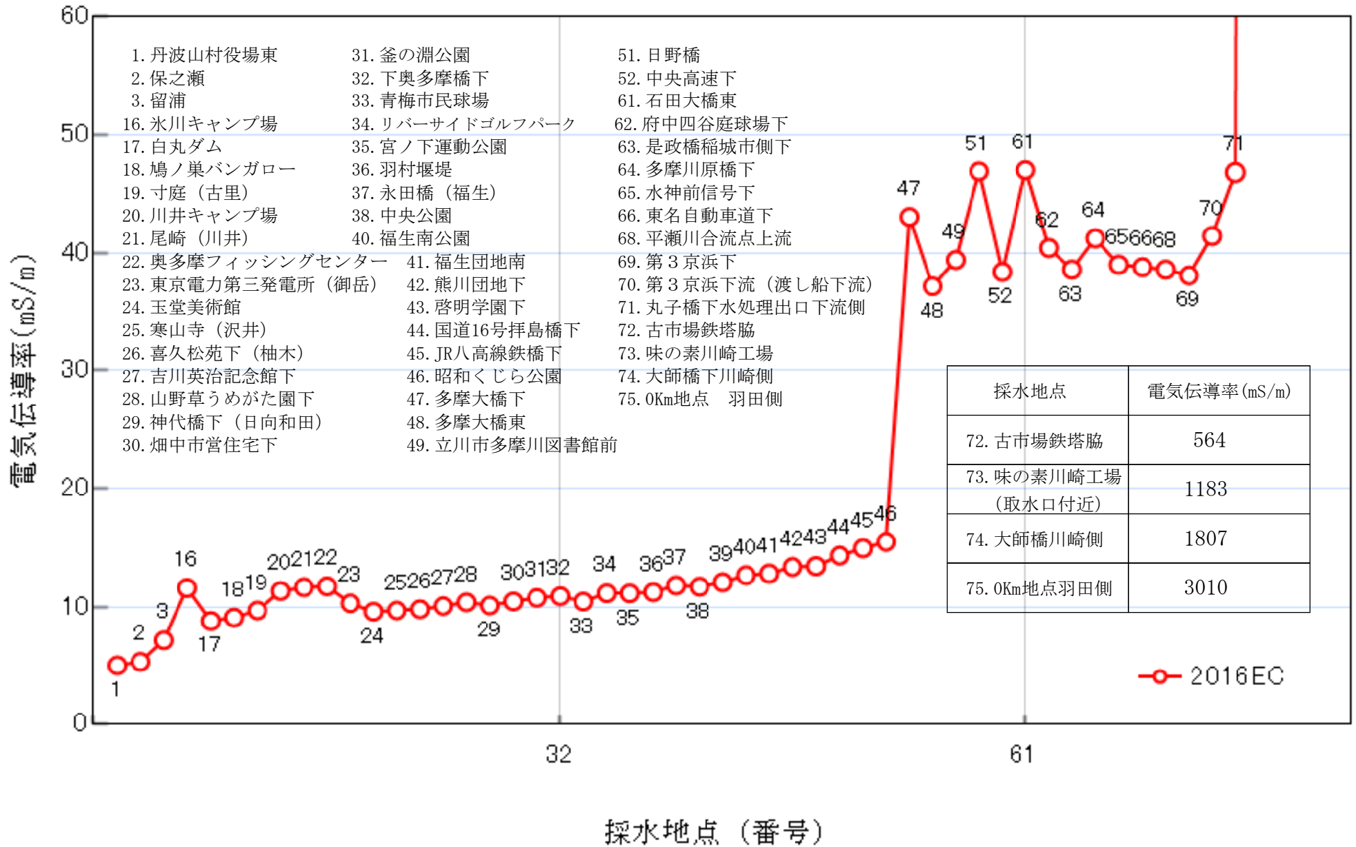
図1 多摩川本川の電気伝導率 (2016. 6. 5)
