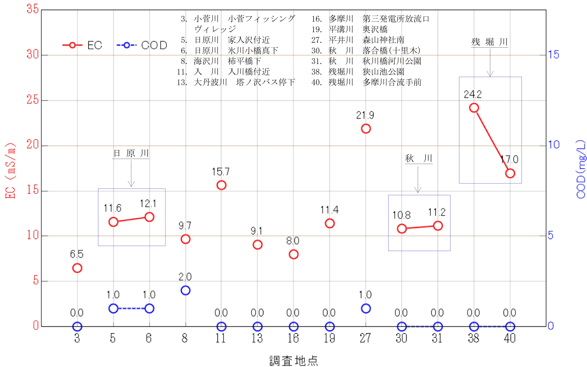
多摩川支川におけるEC・CODの測定結果(2020. 8. 17, 19, 21)
